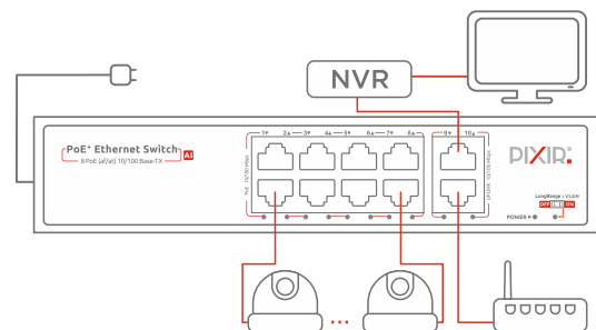
Schemat przykładowego podłączenia PIX-POE8AT-2FE-PS
