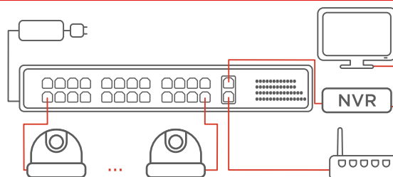
Schemat przykładowego podłączenia PIX-POE24AT-2GE
