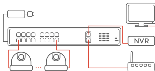
Schemat przykładowego podłączenia PIX-POE16AT-2GE
